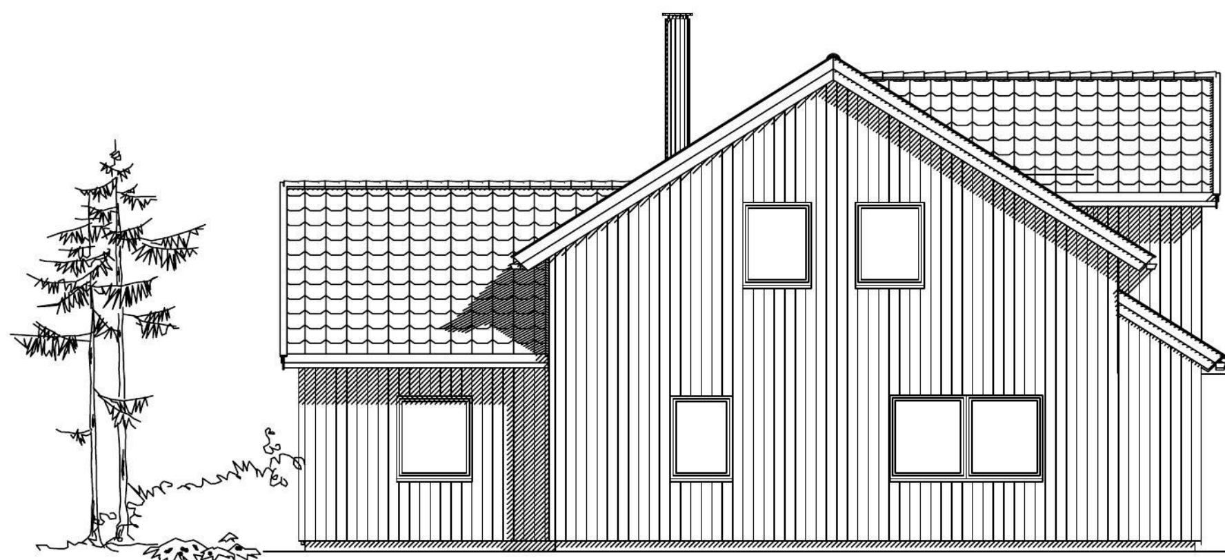
FASADE MOT NORD ØST
